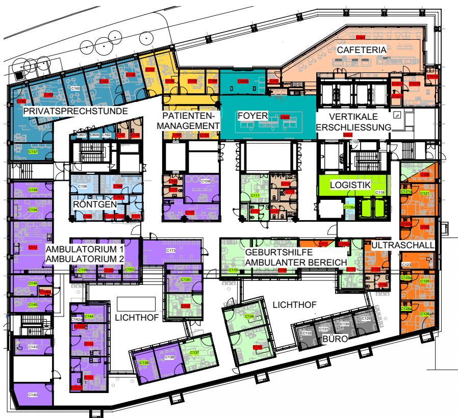
Stockwerkplan Eingangsgeschoss C, Quelle: Inselspital, Insel Gruppe AG
